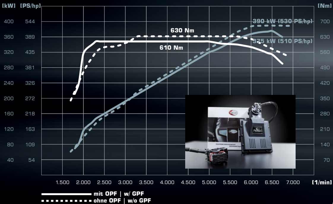
911 Carrera 4S Motor (2019) mit TA 092/S1 Powerkit | 911 Carrera 4S engine (2019) with TA 092/S1 Powerkit
